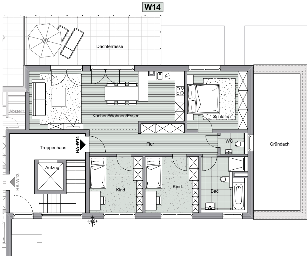
Dachgeschossgrundriss Haus A - W14 M1:100
