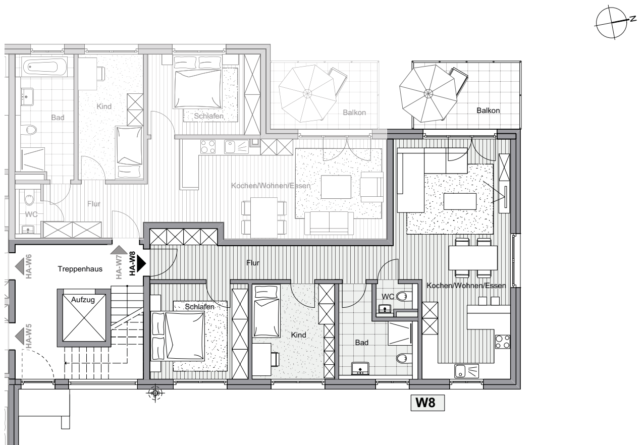
1.Obergeschossgrundriss Haus A - W8 M1:100
